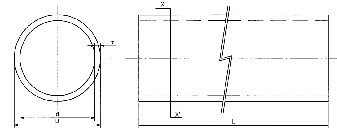
X-X' 断面図
