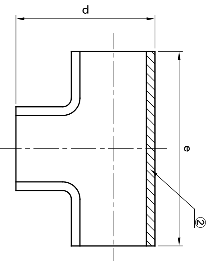
断面図A-A
