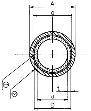
X-X'断面
