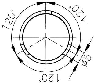
A-A'継手袋ナット断面図
