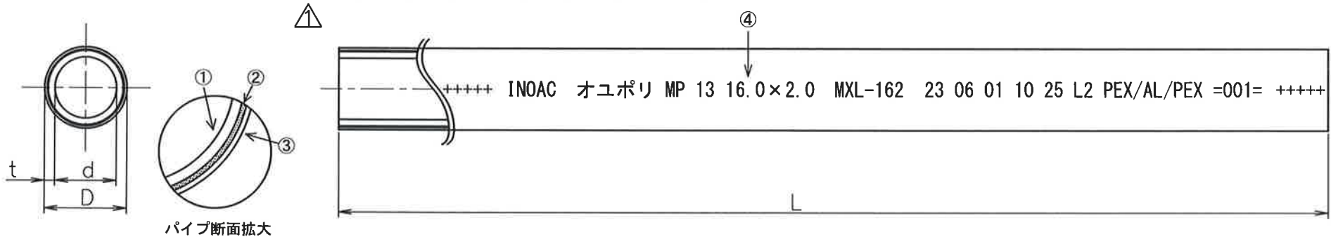
パイプ断面拡大
