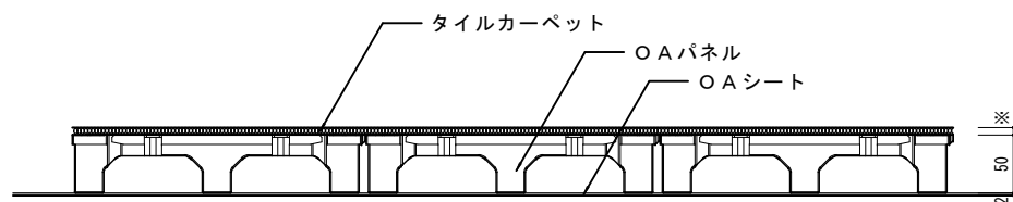
一般中央部断面詳細図 1/5
