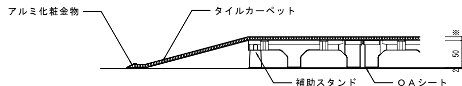
スロープ部分断面詳細図 1/5
