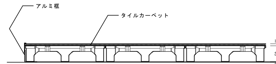
框部分断面詳細図 1/5
