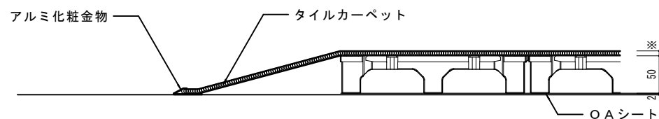
スロープ部分断面詳細図 1/5
