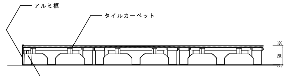
框部分断面詳細図 1/5
