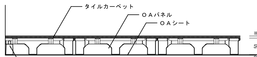
ボーダー部分断面詳細図 1/5
