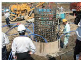
杭利用方式(場所打ち杭)
