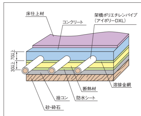
●床構成図
